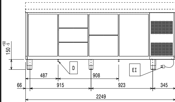
Front aanzicht
